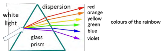
Figur 1.3: Vitt ljus delas upp i sina beståndsdelar genom refractionen (brytningen) i en glasprisma (tack till PNGImage).
