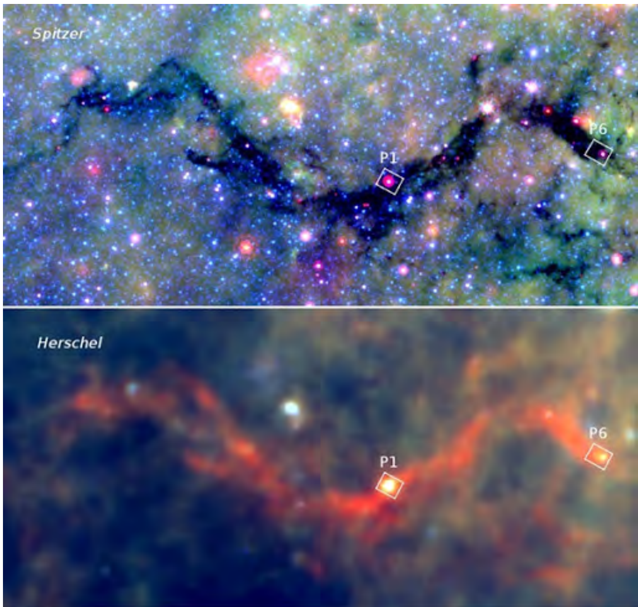
Figur 1.8: Ett exempel på ett tätt interstellärt molekylnmoln, kallat "Ormen". Den övre bilden är tagen med rymdteleskopet Spitzer vid rätt korta infraröda våglängder. Ormen är så tät och innehåller så mycket stoff att dessa infraröda våglängder absorberas av molnet, och vi ser det som en mörk skugga. Sådana ting som Ormen kallas " infraröda mörka moln " (på engelska Infrared Dark Clouds, IRDCs ), och vi ska studera dem som exempel på moln i vilka stjärnor just har börjat bildas, såsom objekten "P1" och "P6" som har markerats. Den nedre bilden visar samma område på himlen, men nu sett i längre infraröda våglängder med rymdteleskopet Herschel. Se hur Ormen nu glöder kraftigt eftersom dess kalla stoff strålar starkt i dessa våglängder (tack till Jean-Charles Cuillandre).
