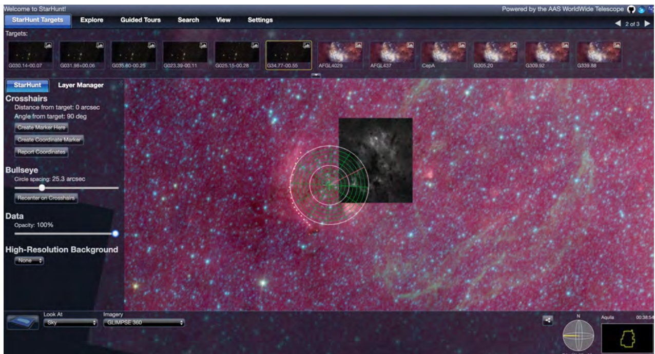
Figur 3.11: Ett exempel på bubbla som hittats runt molekylnmolnet G034.77-00.55. Femettan ligger på mitten av bubblan och har utvidgats till en radie motsvarande bubblans. Formen på bubblan visas av gula markörer.
