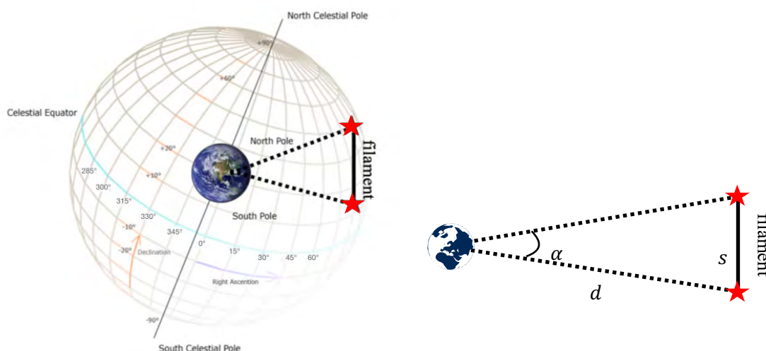
Figur 3.10: Till vänster: Himmelssfären med jorden i mitten. Himmelsekvatorn och norra himmelspolen är angivna. De röda stjärnorna visar ändarna av ett filament på himmelssfären. Bild: Lone Wolf online. Till höger: En skiss av triangeln som bildas av filamentets ändar och jorden. Vinkelavståndet \alpha , den fysiska storleken s och avståndet mellan filamentet och jorden, d , är angivna.
