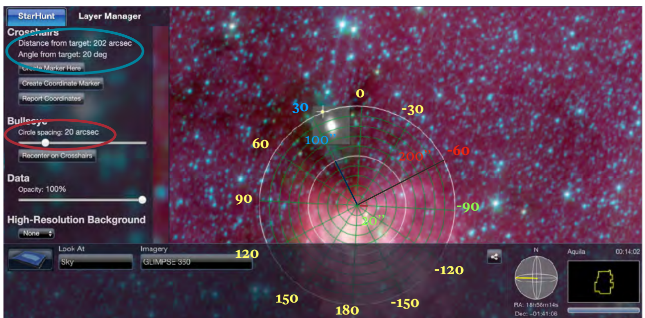
Figur 2.3: Demonstration av markör och bullseye-verktyget (femettan). Lägg märke till att vi har ändrat bakgrunds bilden (2MASS och GLIMPSE). Markören visas som en gul prick. Dess avstånd och vinkel från femettans mitt är inringade i båda bildernas övre vänstra hörn.
